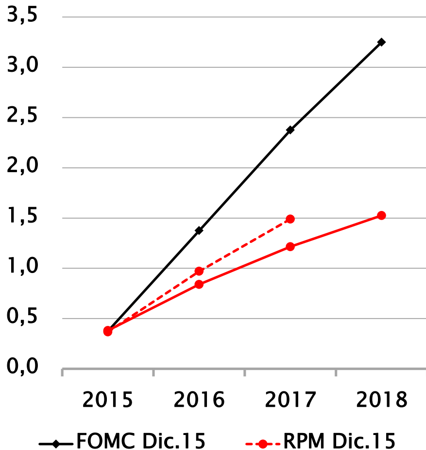
EE.UU: Trayectoria Fed fund
