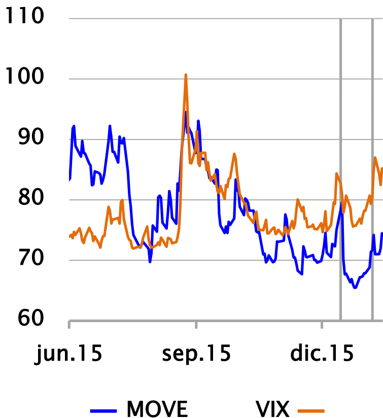
MOVE y VIX (1) (puntos base; porcentaje)
